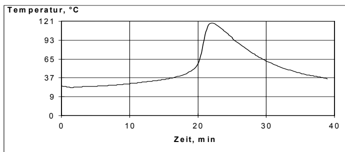
Typische Reaktivitätskurve für MA310 at 23°C (10 grams) 5
